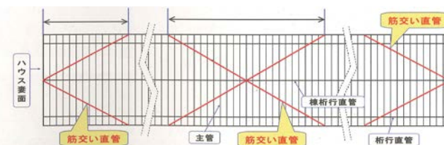
筋交いによる妻面の補強方法事例
