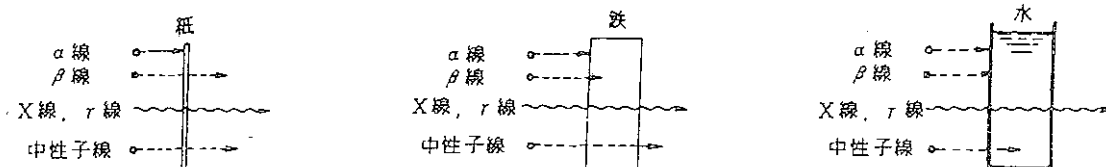
図 8 放射線の吸収
