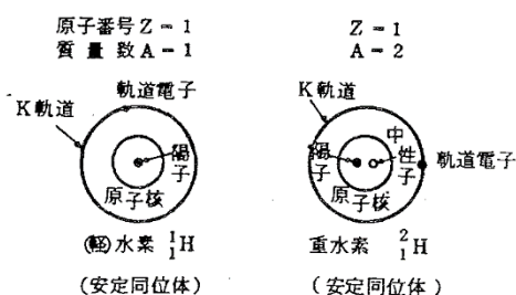
図4 水素の同位体と原子の構造
