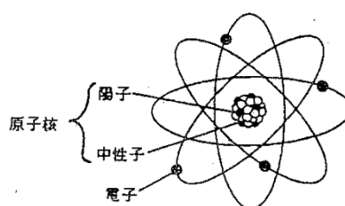
図2 原子の構造
