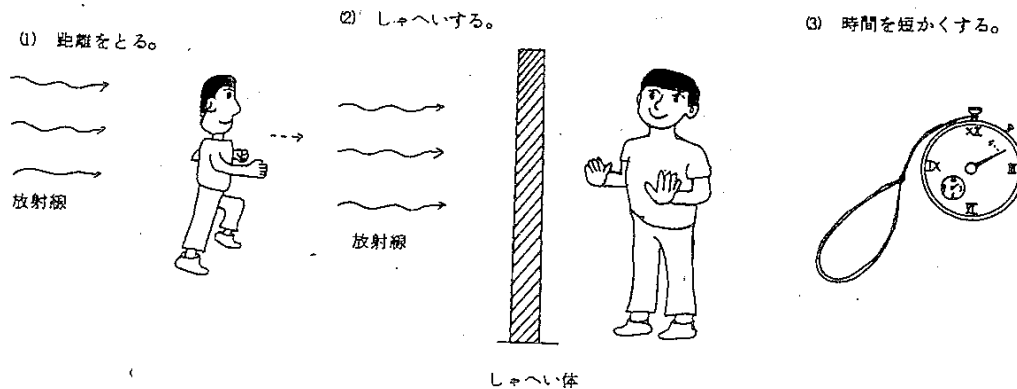
図10 外部被ばく防護方法の3原則
