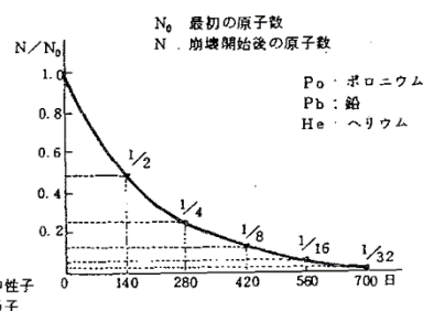
図6 半減期
