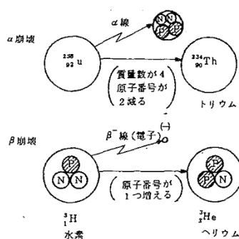
図5 原子核の崩壊
