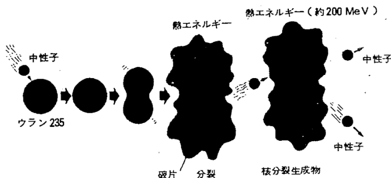
図7 核分裂
