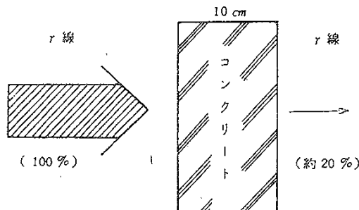
図11 コンクリートのしゃへい効果
