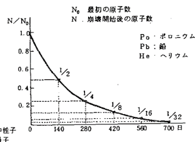
図6 半減期
