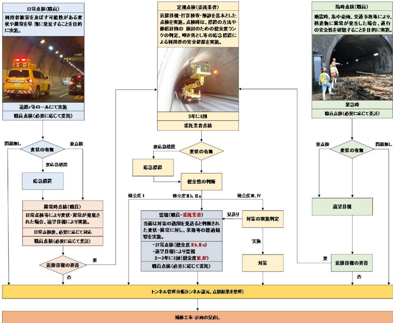
図 3.2.1 点検体系のフロー
