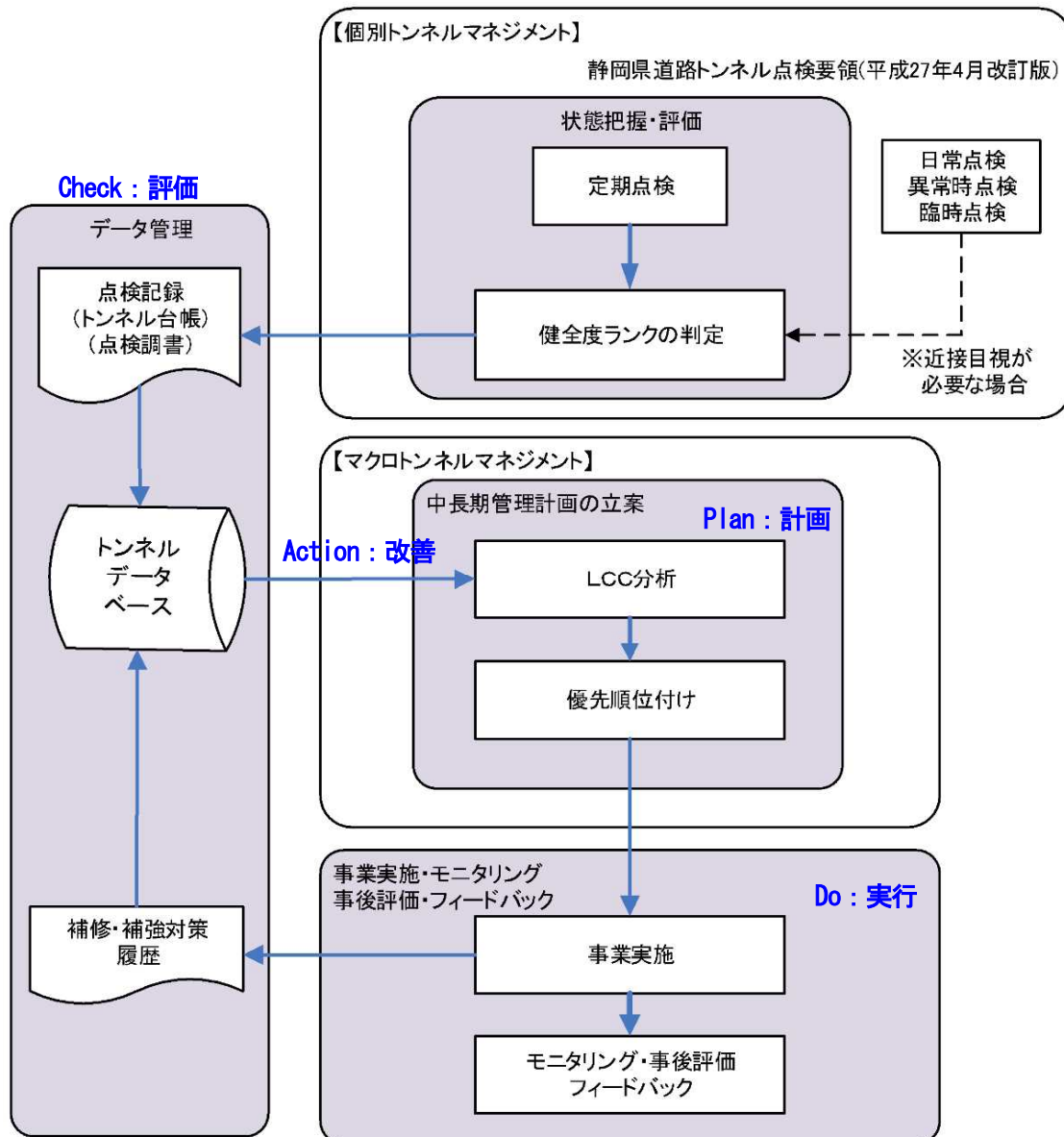
図 1. 2. 1 トンネルマネジメントの体系
