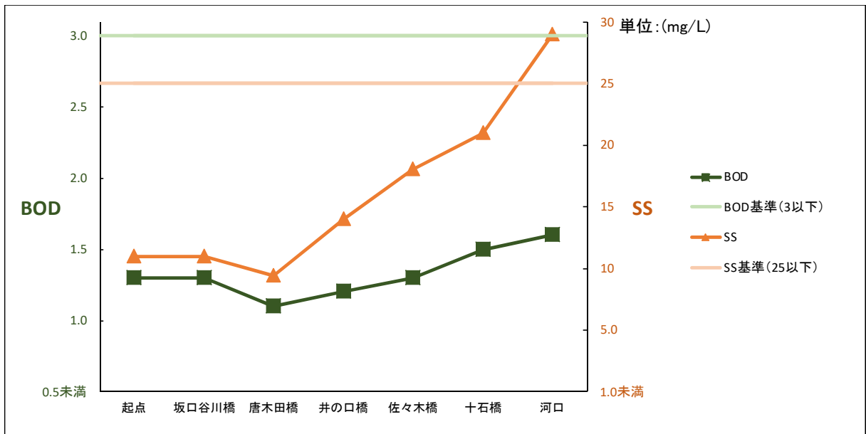
図 1-1-2 BOD(mg/L)、SS(mg/L)
