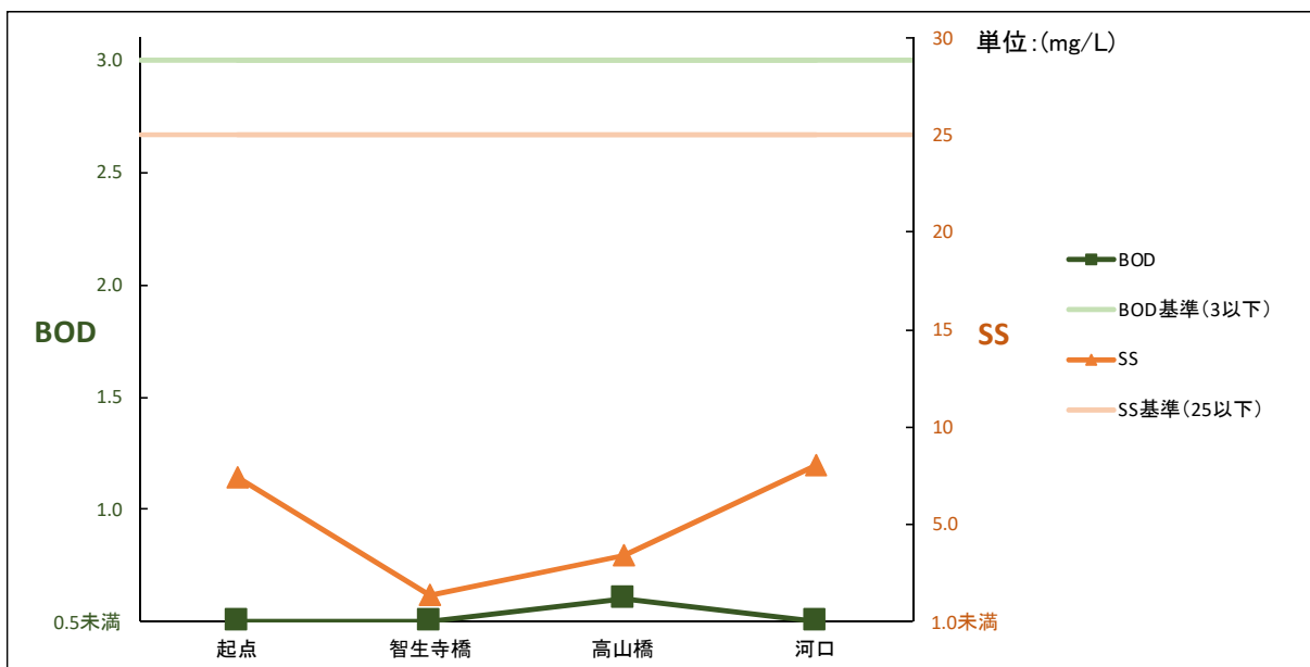
図 1-2-2 BOD(mg/L)、SS(mg/L)
