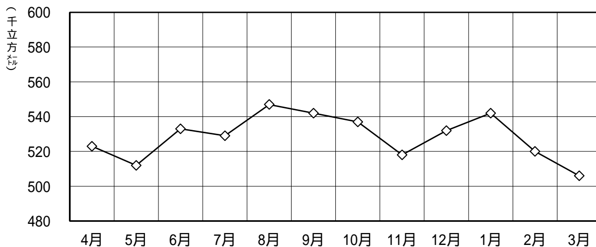
令和2年度 月別配水量
